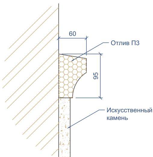
Разрез 5-5
