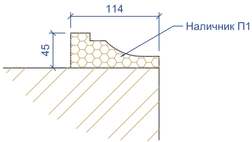
Сечение 1-1
