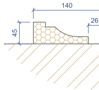
Сечение 2-2
