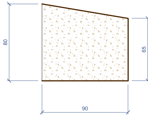
Вид слева (Масштаб 1:2)
